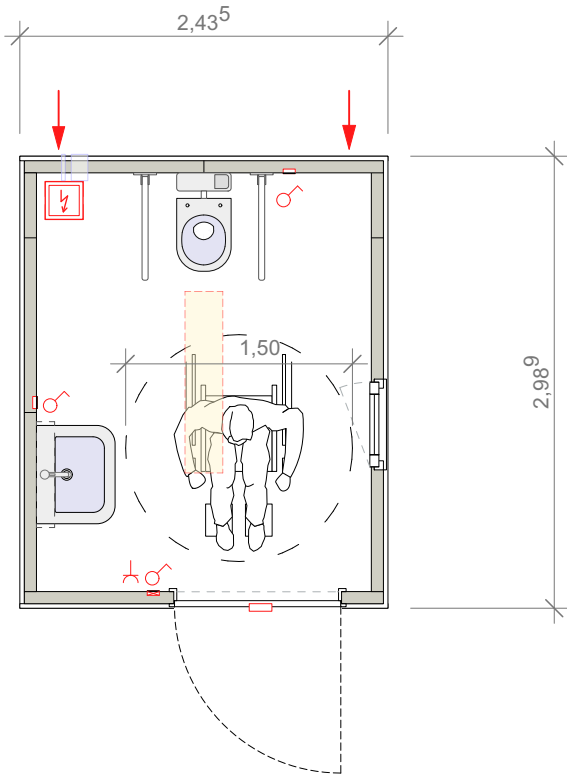
C-Tec-600-barrierefrei
